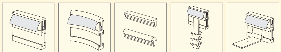
Grundprofil mit Klemmschiene flach Grundprofil mit Klemmschiene rund Folienklemmschienen (für Folien bis 0,5 mm) Beton-/Erdanker 90°-Profilanker
